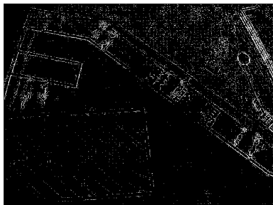
図5 二値化画像
